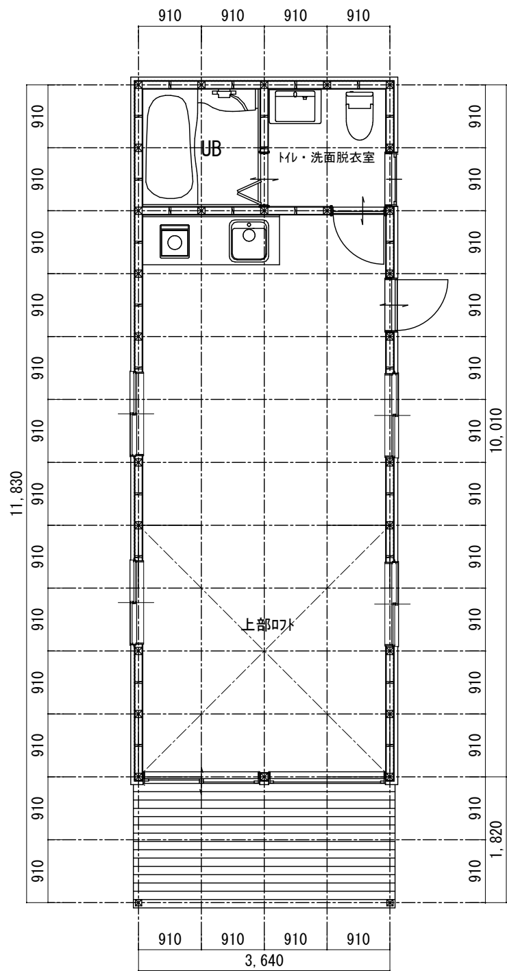
平面図 S=1/75
