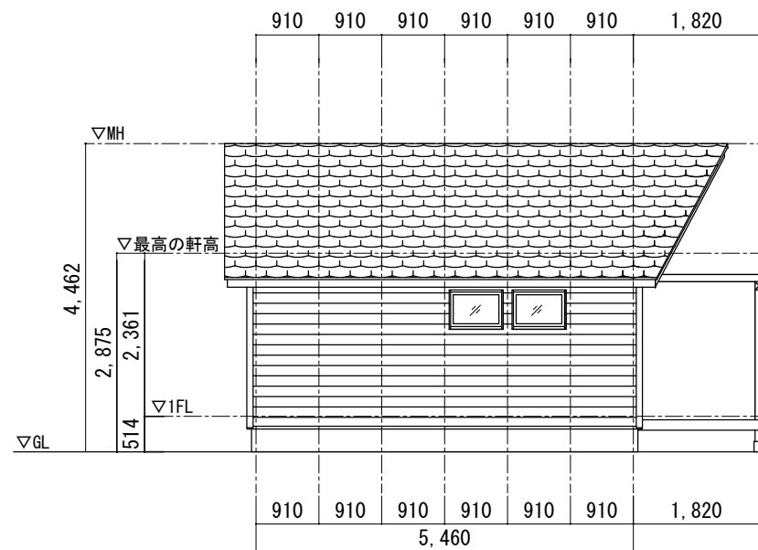
D面立面図 S=1/100
