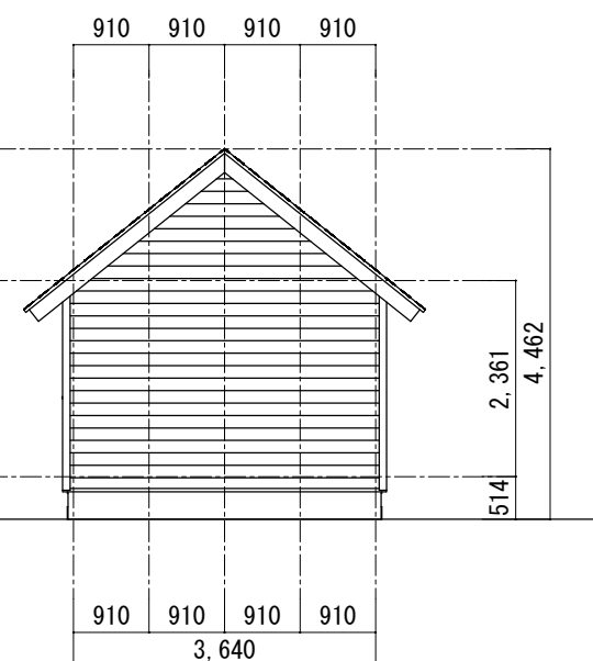
A面立面図 S=1/100
