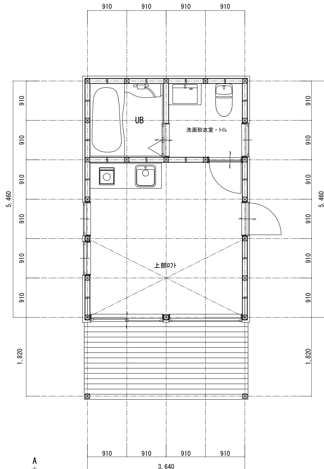
平面図 S=1/50
