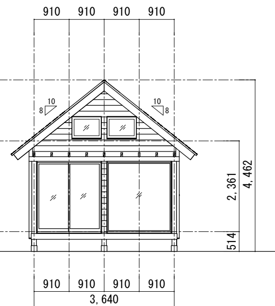
C面立面図 S=1/100
